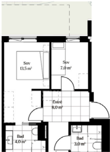
Alternativ planløsning
