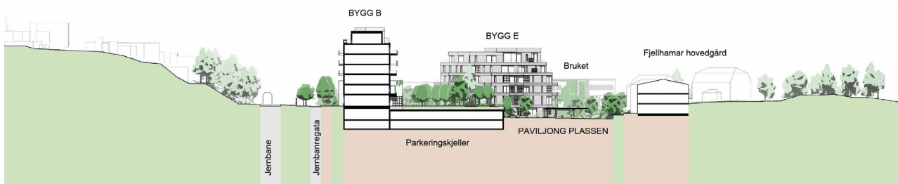
Snitt gjennom Østfeltet. Ill: SOLA/Code
