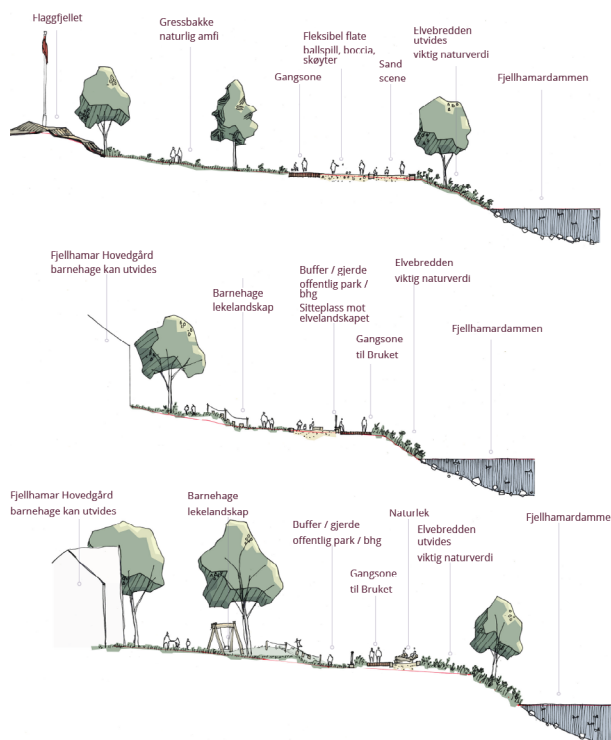
Illustrasjonssnitt Flaggfjellparken. Ill: SOLA
