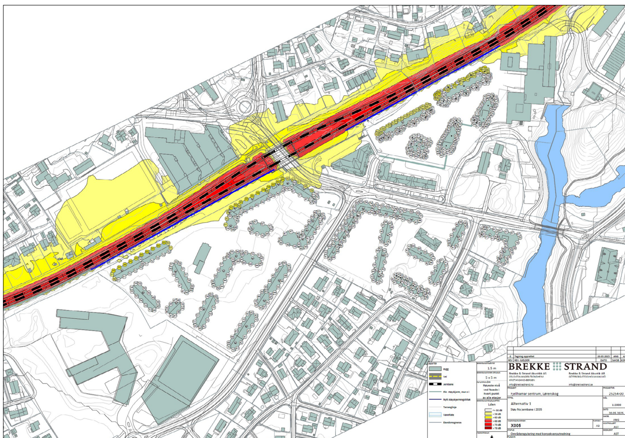
5.13 Støy fra jernbane. Blå tykk strek viser støyskjerm langs jernbane. III: Brekke & Strand
